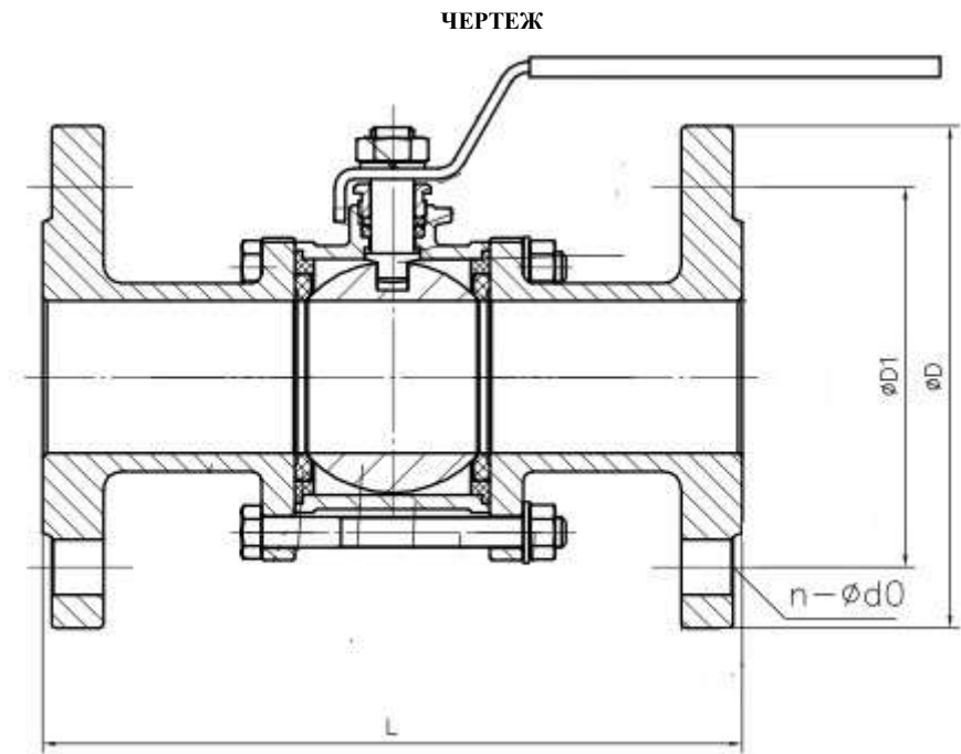
ГАБАРИТНЫЕ И ПРИСОЕДИНИТЕЛЬНЫЕ РАЗМЕРЫ
